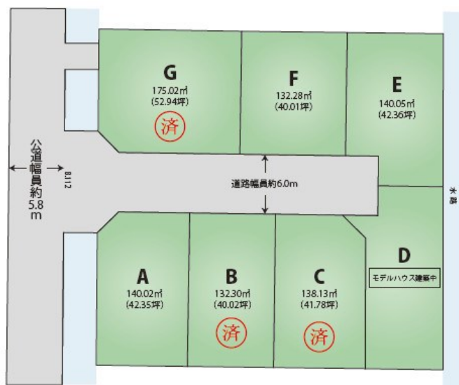
■ 区画図
